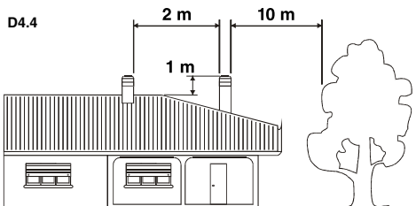
(1) La chimenea no debe tener obstáculos en un espacio de 10 m desde paredes, faldas y árboles. De lo contrario, elevar la misma como mínimo 1 m sobre el obstáculo. La chimenea debe superar la cumbre del tejado en 1 m como mínimo.
