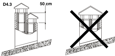
(1) En caso de conductos de humos colocados uno al lado de otro, uno deberá superar al otro como mínimo en 50 cm, para evitar traslados de presión entre los mismos.
